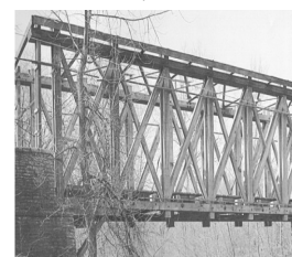
Pont en bois (Brownsville TEXAS)
