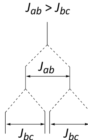
Multiplet mal défini
